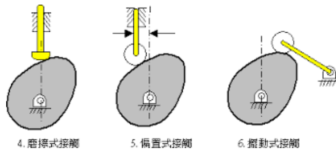
常見凸輪機構的概念圖
